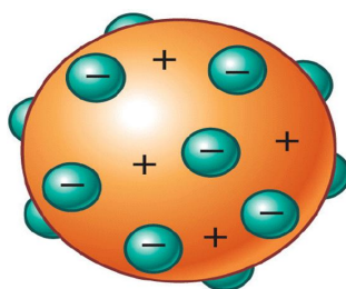
Figura 4: Átomo de Thomson
