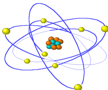
Figura 5. Átomo de Rutherford
