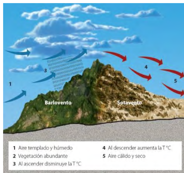
Figura 32: Representación gráfica del proceso de formación del efecto Föhn
