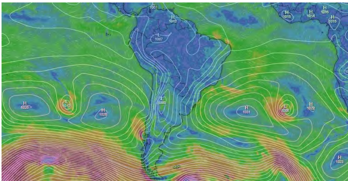
Figura 27: Representación de Isobaras. Centros de alta (H) y baja presión (L)
