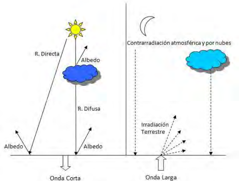
Figura 14: Flujos energéticos y tipos de radiación: onda corta diurna y onda larga nocturna
