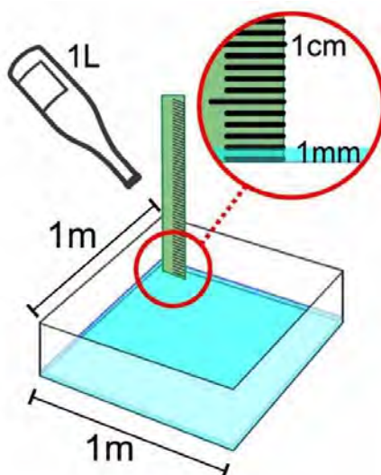
Figura 47: Representación gráfica de lo que equivale 1 mm de precipitación
