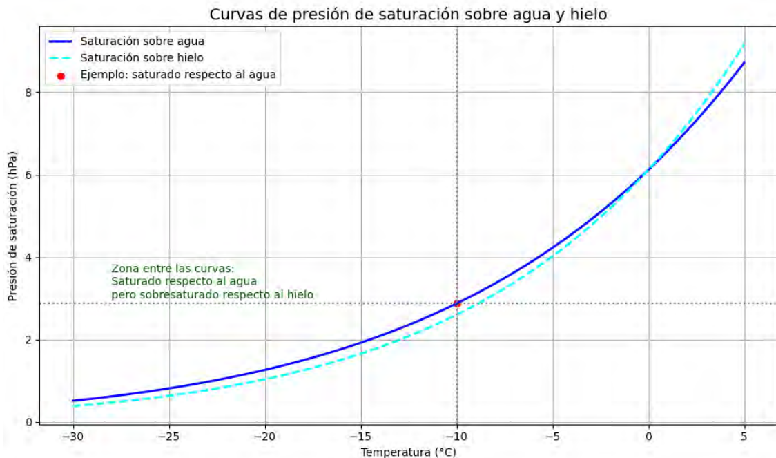
Figura 46: Gráfica de la curva de saturación por debajo de cero grados
