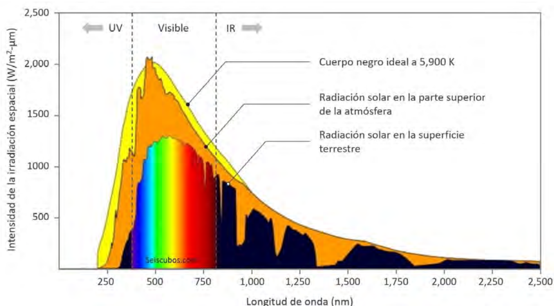
Figura 9. Espectro solar
