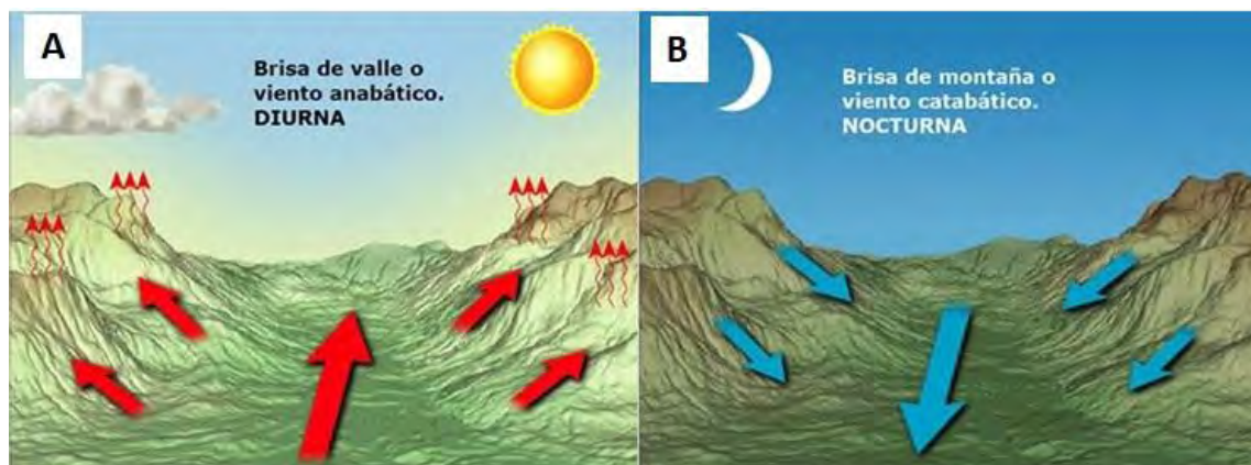
Figura 30: Circulaciones periódicas locales. A-Brisa de valle. B-Brisa de montaña Fuente: Tomado de Brisas: los vientos que te refrescan por Llorente (2018)
