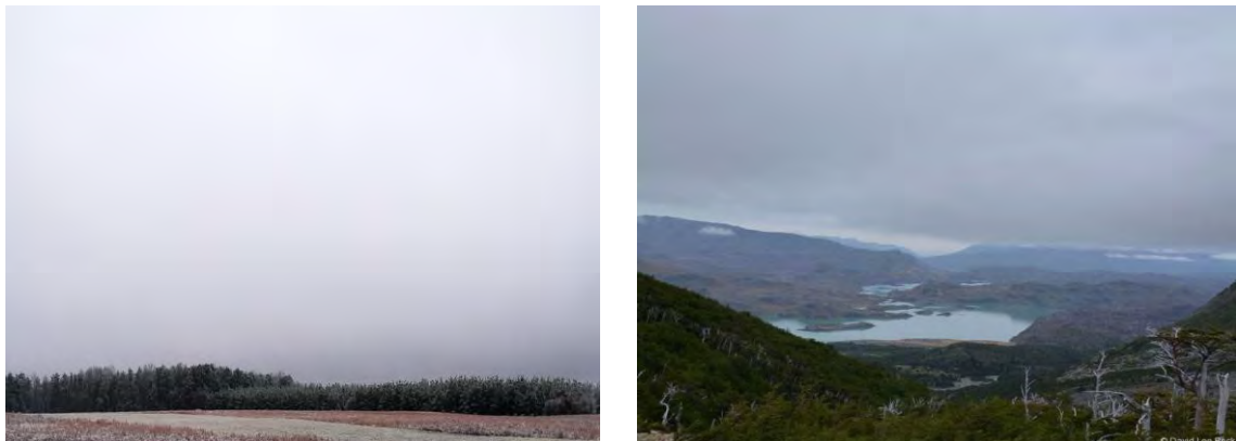
Figura 42: Nubes Stratus, con aspecto uniforme y grisáceo, típica de mañanas nubladas o condiciones de alta humedad.
