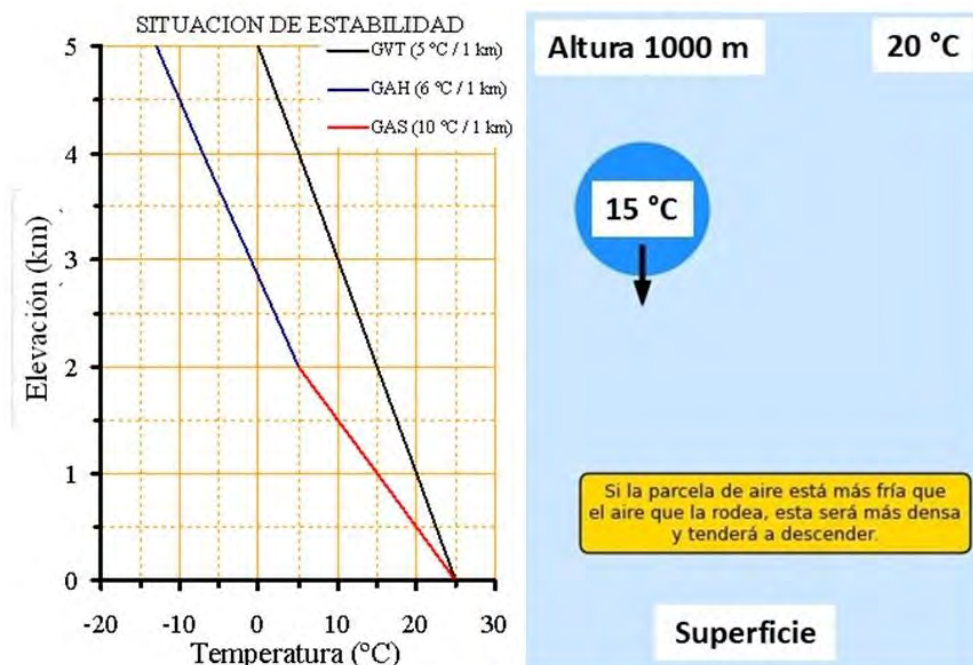
Figura 20: Situación de atmósfera estable
