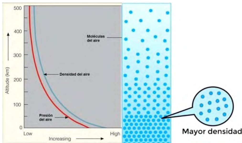
Figura 4. Gráfica de la variación de la presión y la densidad del aire con la altura
