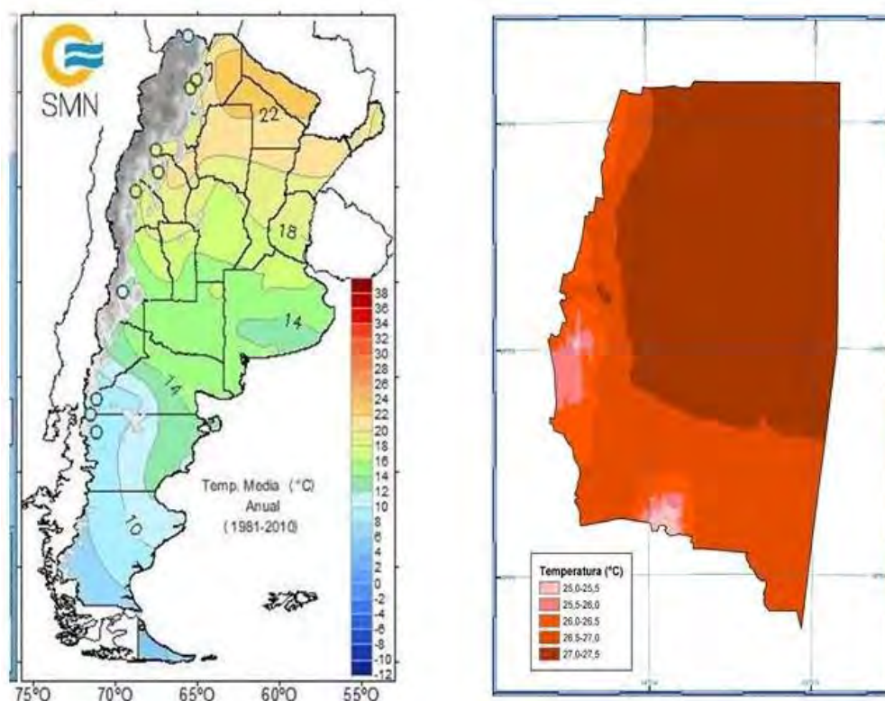
Figura 24: Tendencia de isotermas medias anuales en Argentina y del mes de enero en Santiago del Estero.
