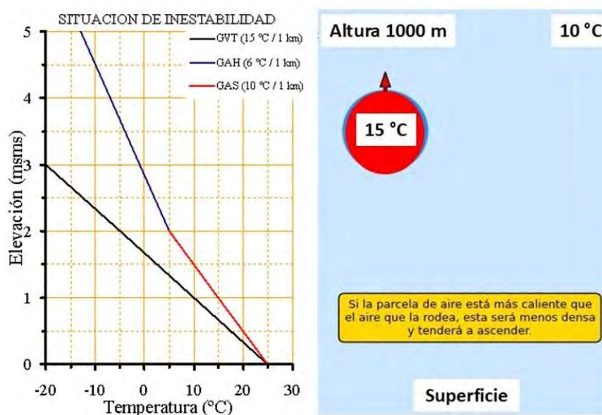
Figura 21: Situación de atmósfera inestable
